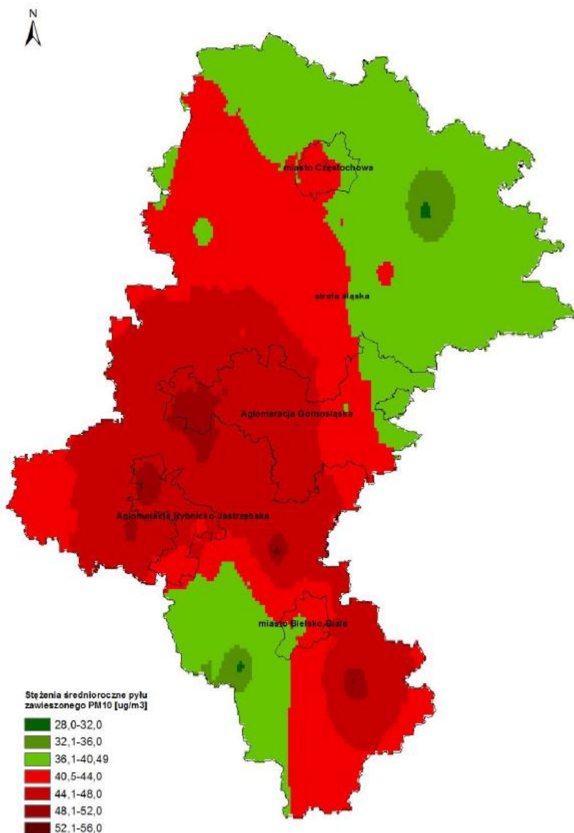
Rysunek 2-19 Obszary przekroczeń średnich stężeń rocznych pyłu zawieszzonego PM10 - kryterium ochrona zdrowia ludzi
