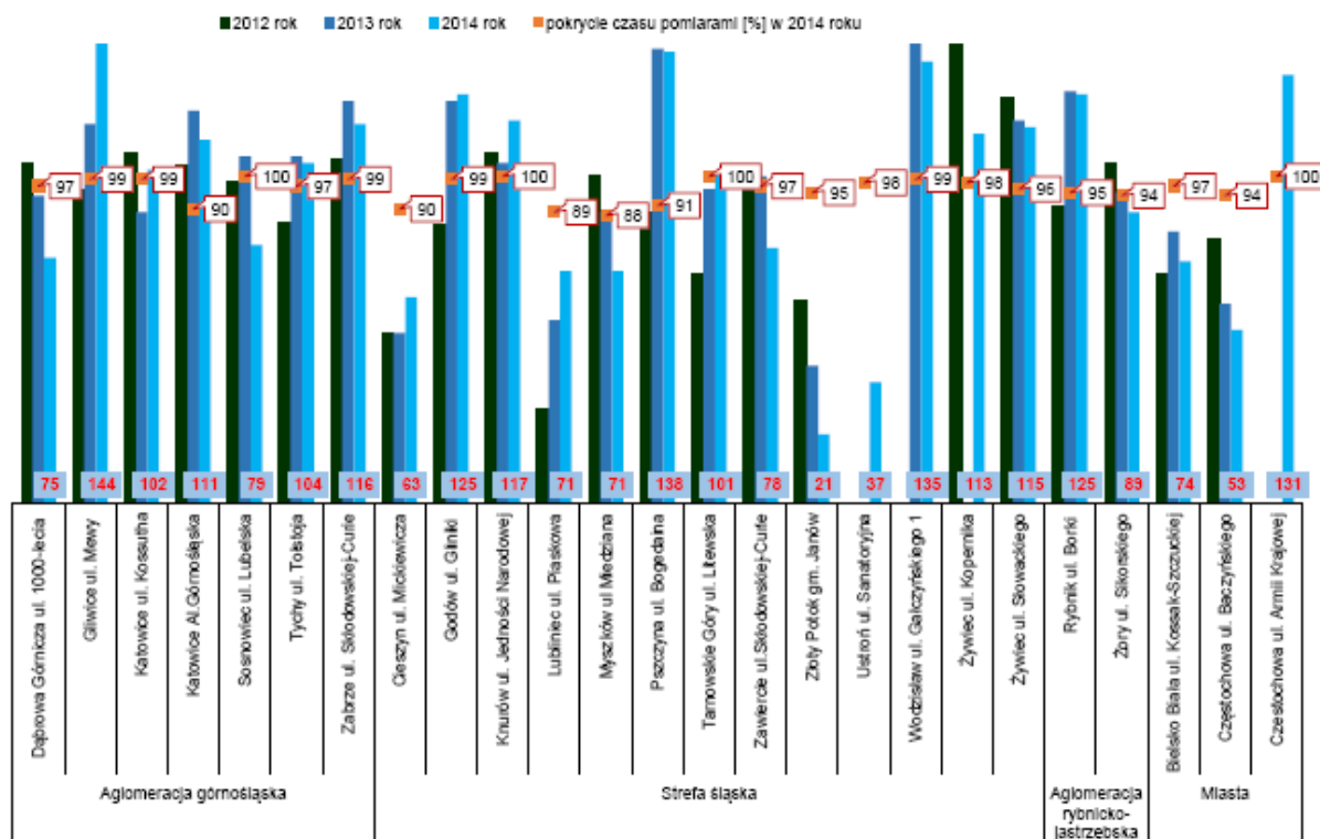
Rysunek 2-23 Liczba przekroczeń dopuszczalnego poziomu stężeń 24-godzinnych pyłu zawieszzonego PM10 w latach 2012-2014 (wartości w etykietach dot. 2014 roku) oraz pokrycie czasu pomiarami w procentach w 2014 roku
